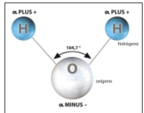
La estructura química de una molécula del agua
